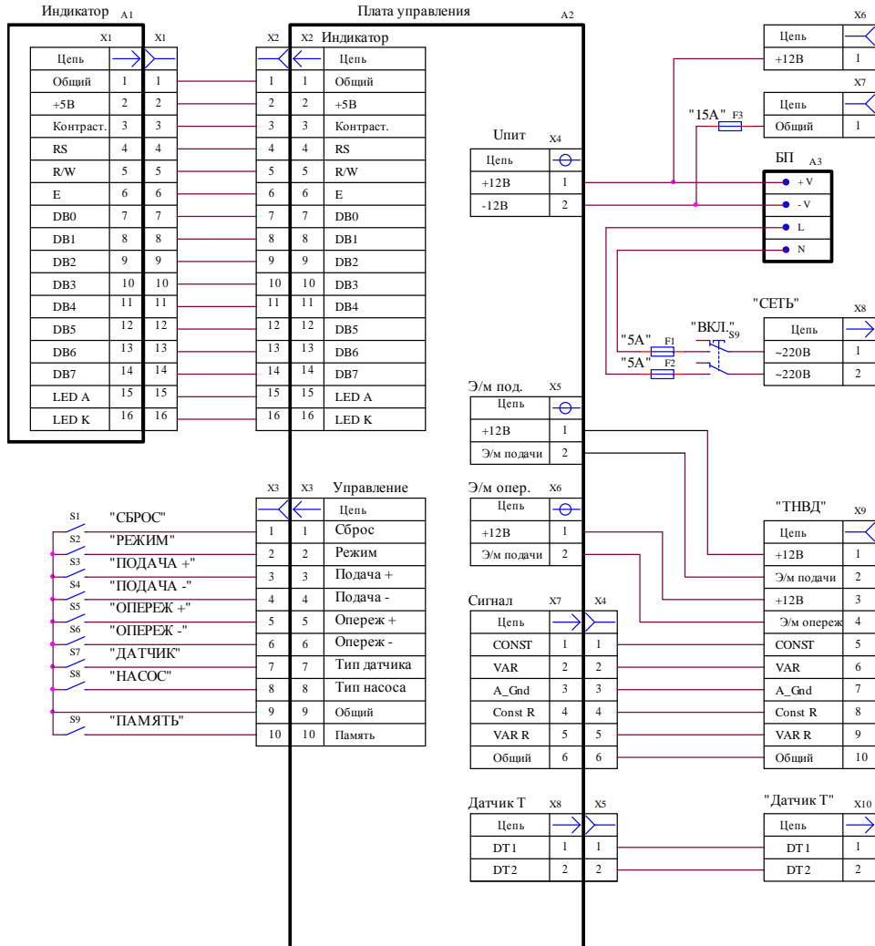
Контроллер КТН-2М. Схема электрическая общая
