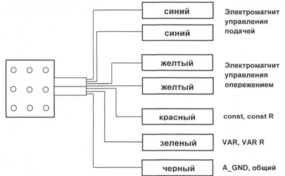
Кабель соединительный
